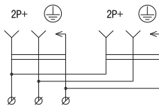
Рисунок 3 – Электрическая схема соединений РБ32-1-0м
